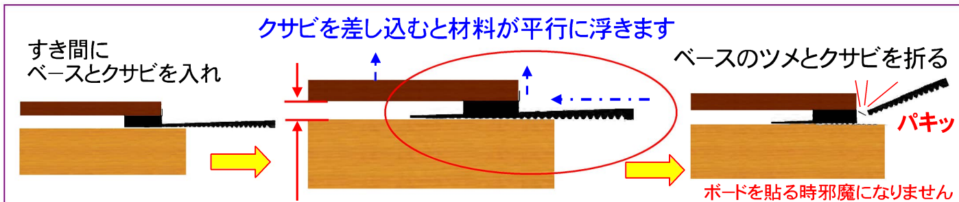
調整クサビ120
